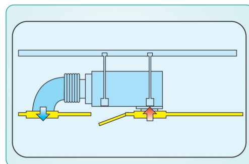
Воздухозабор снизу (схема 1)
