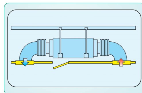
Стандартный воздухозабор (схема 2)
